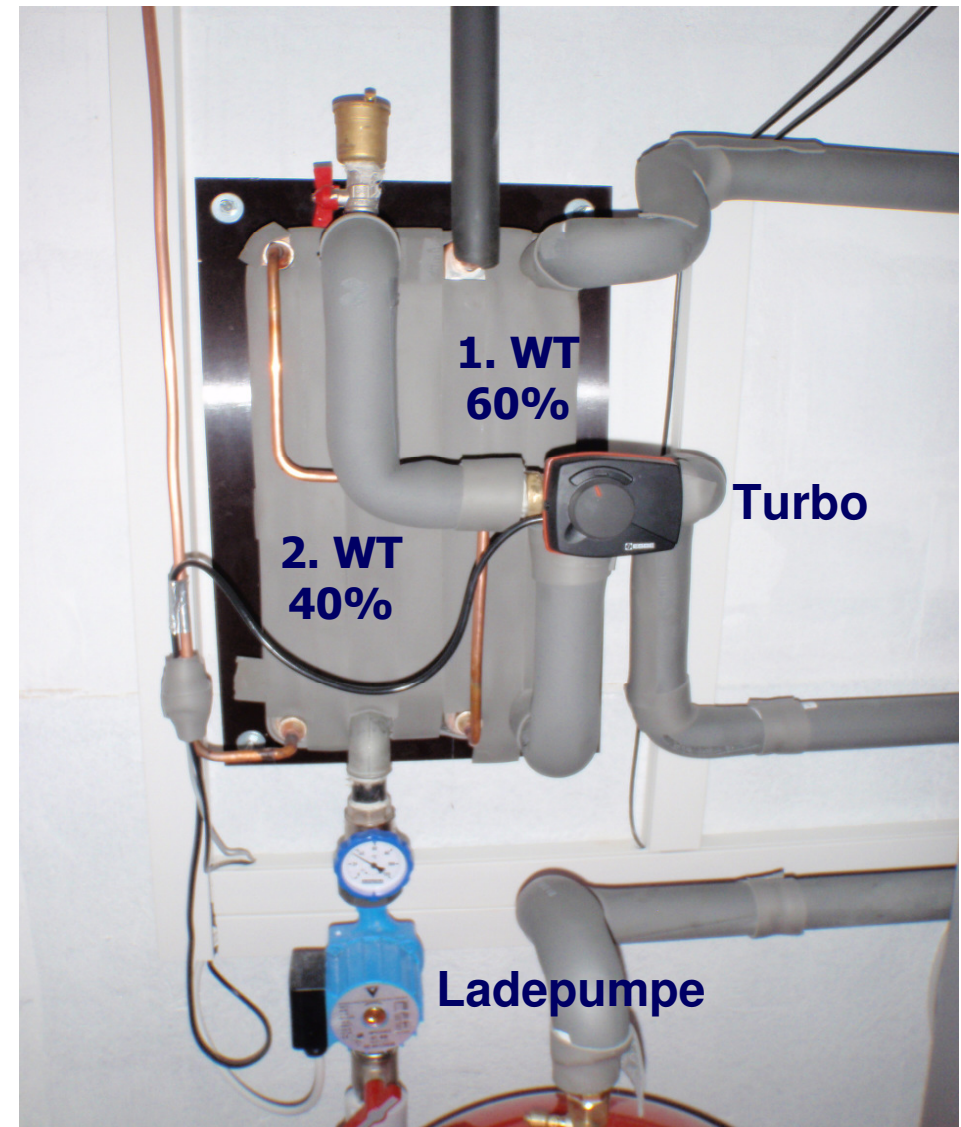
Kompaktstation: „Hydro-Turbo-Box“
